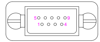
视图A(航插) 1:5
